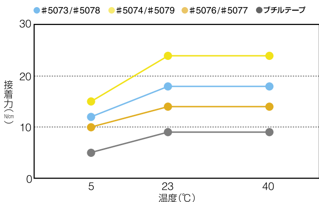
霧気温度別 貼り付け直後(30秒後)接着性(90°C剥離強度)
