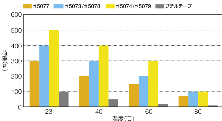
霧気温度別 剪断保持力(テープサイズ:10mm×25mm)
