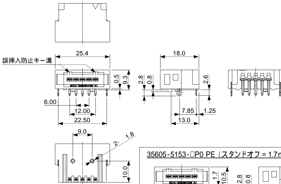
35605-5153-□00 PE (スタンドオフ = 0.5mm) 外形図
