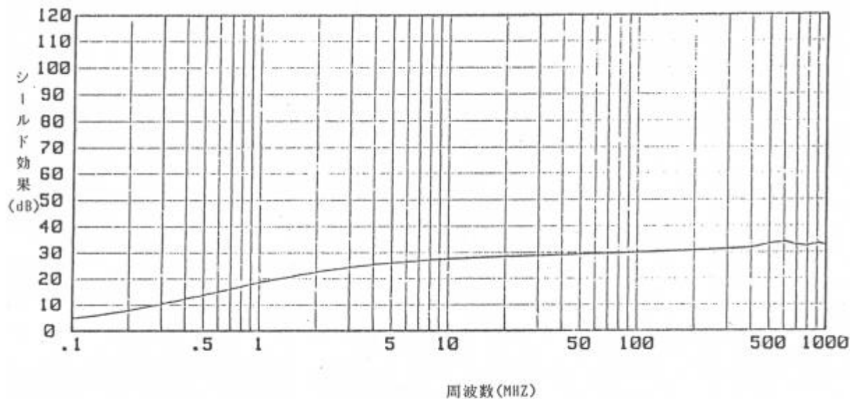
図-3.KEC法による#1170のシールド効果
