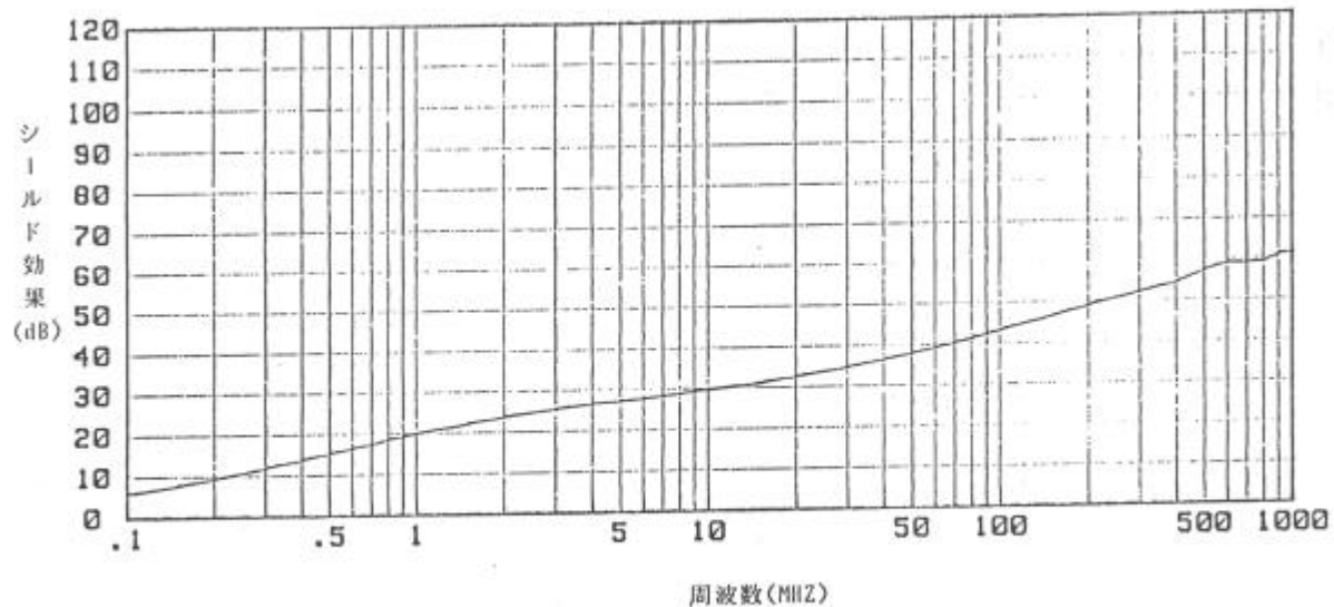
図-3.KEC法による#1181のシールド効果
