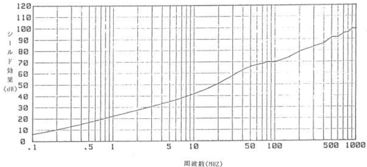
図-3.KEC法による#1245のシールド効果
