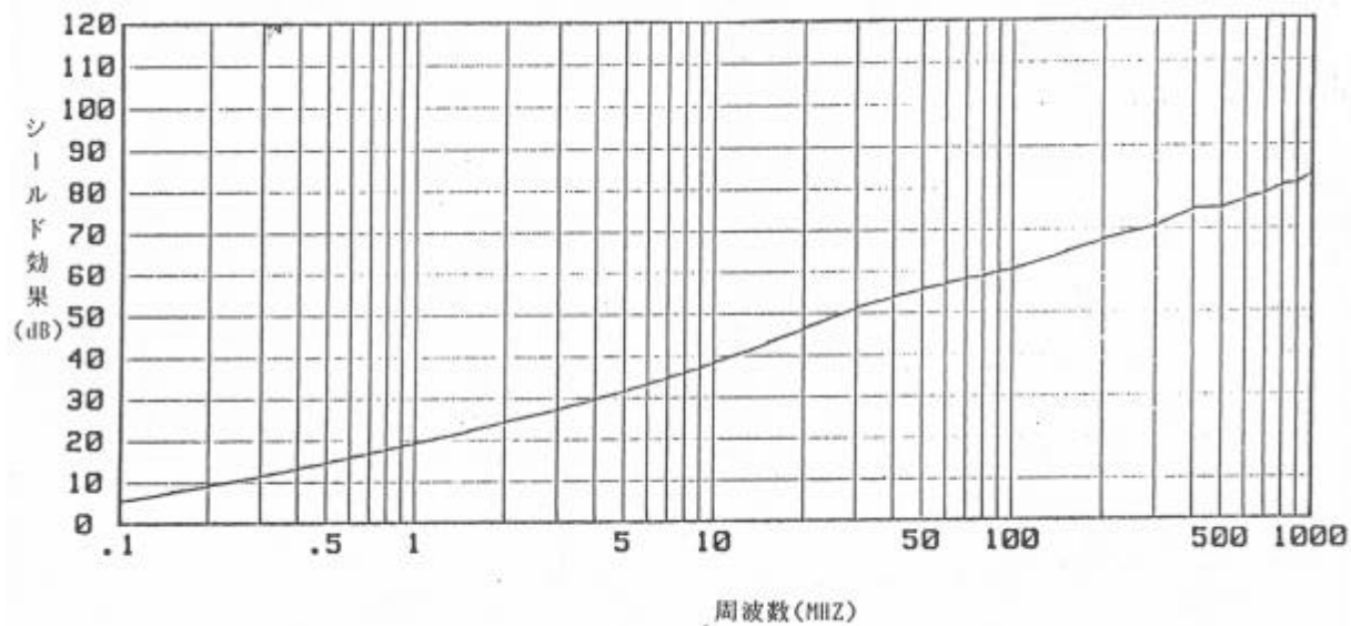
図-3.KEC法による#1267のシールド効果
