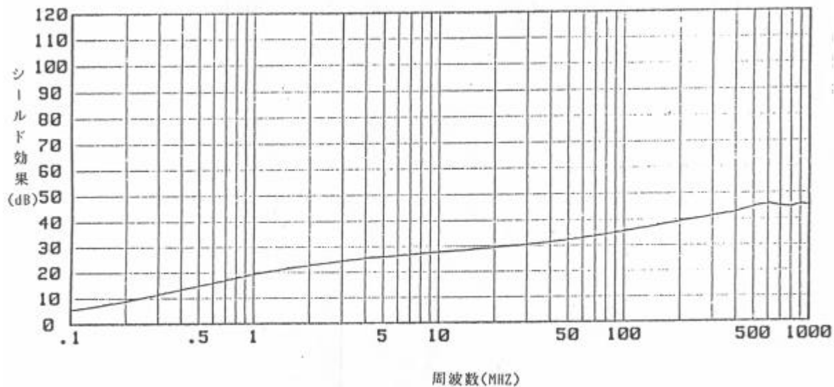
図-3.KEC法による#2245のシールド効果
