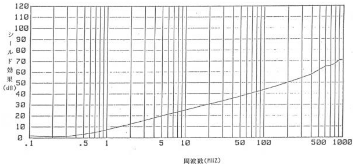
図-3.KEC法によるAL-35FRのシールド効果
